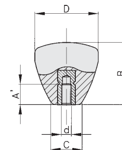
insert taraudé en acier zingué * laiton dans référence 2271
