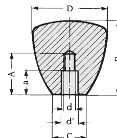
taraudage moulé, avec chambrage
