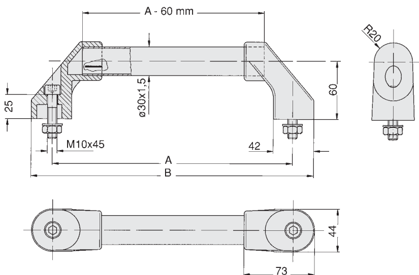
Poignée avec tube diamètre 30 mm, livrée assemblée, avec fixations
