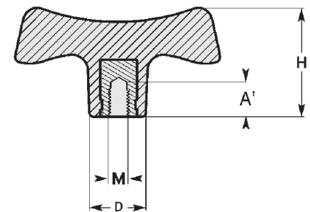
insert taraudé en acier zingué
