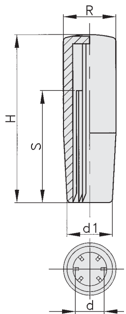
trou lisse intérieur avec cannelures
